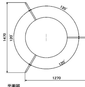
平面図
