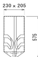
バルーン部収納時
